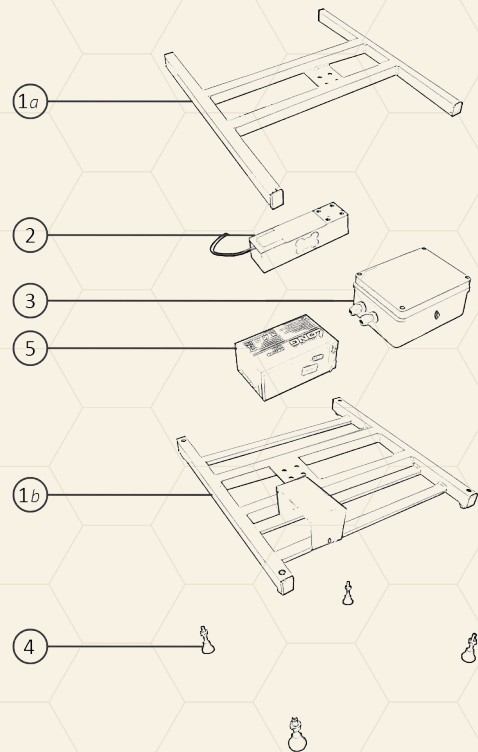
Abbildung 2. Hauptteile der SMS-Waage
