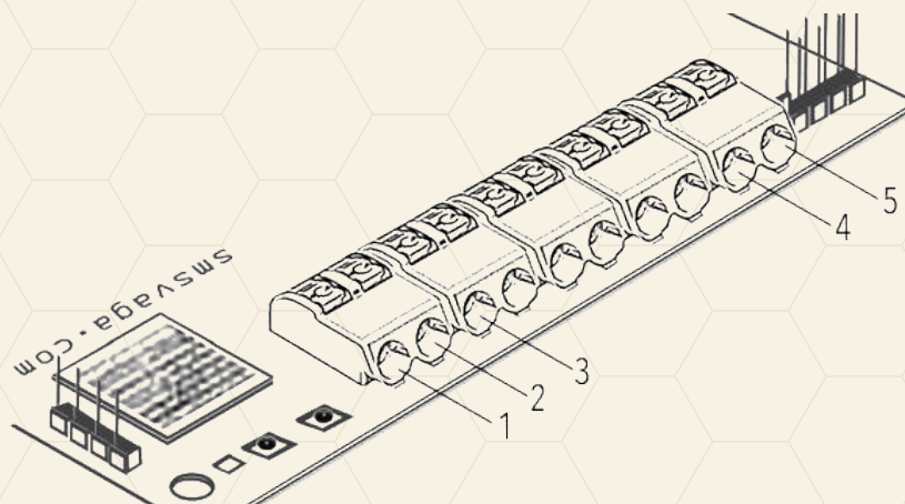
Abbildung 4. Anschließen der Sensoren
